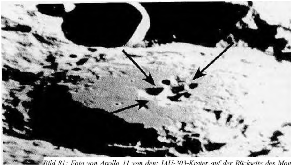
Bild 81: Foto von Apollo 11 von den: IAU-303-Krater auf der Rückseite des Mondes.
