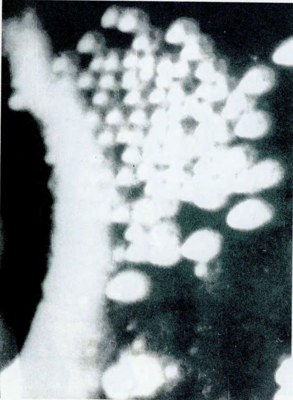
Bild 58: Foto von NASA Lunar Orbiter V, Ni: MR 82, Teil des Kraters Ritter C. Kegelförmige Wolken und Kumuluswolken.
