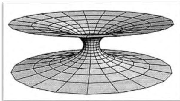
Fig 2-6. Einstein-Rosen Bridge.
